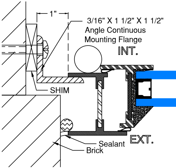
#1 BRICK -FLUSH
